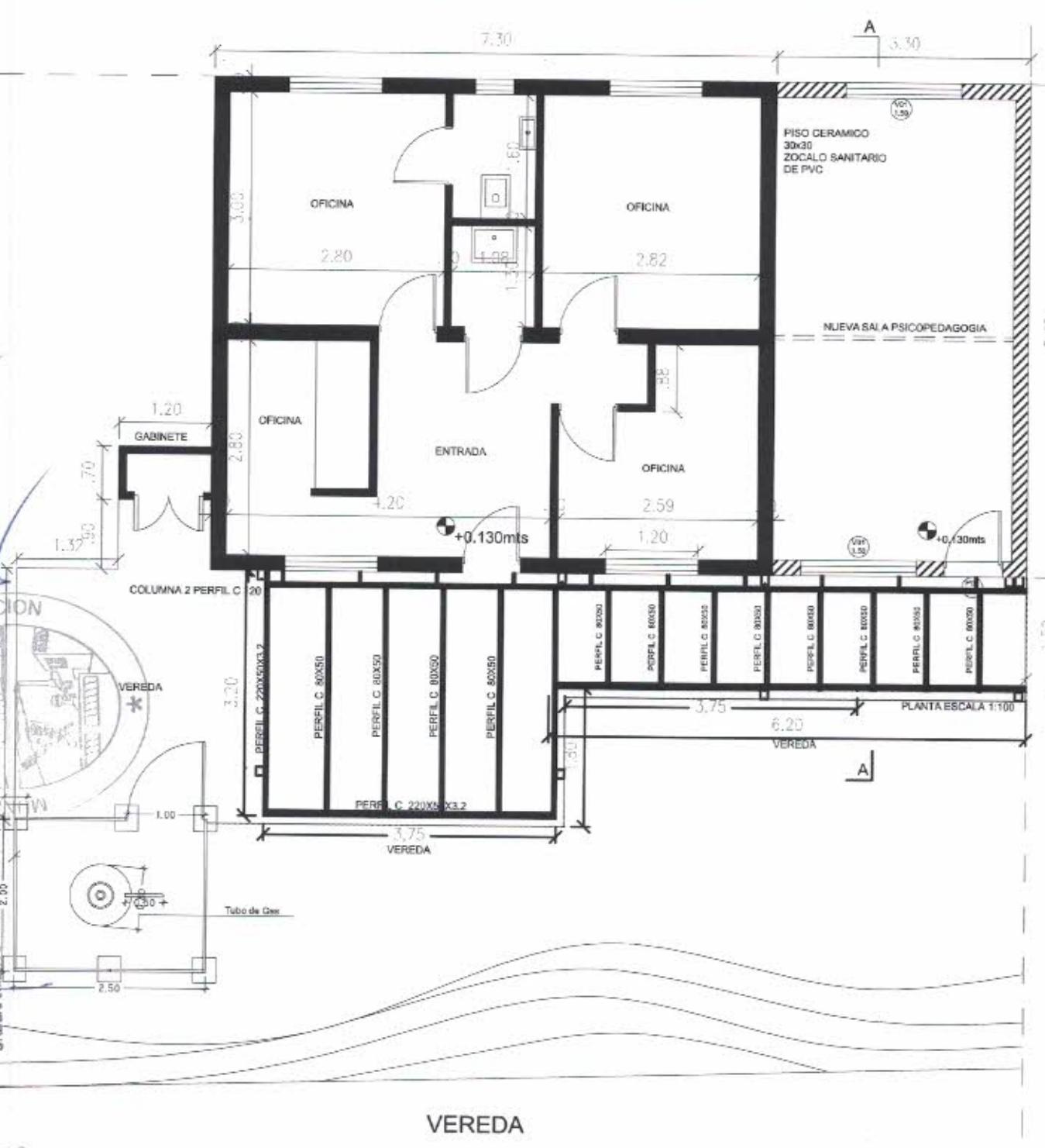
PLANO OBRA NUEVA
